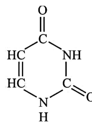
Uracil (U)
