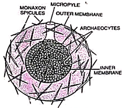
Fig. 1.13. Gemmule
